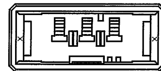
X キーイング パターン X KEYING PATTERN 1-178802-3 ONLY
