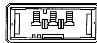
Y キーイング パターン Y KEYING PATTERN 2-178802-3 ONLY
